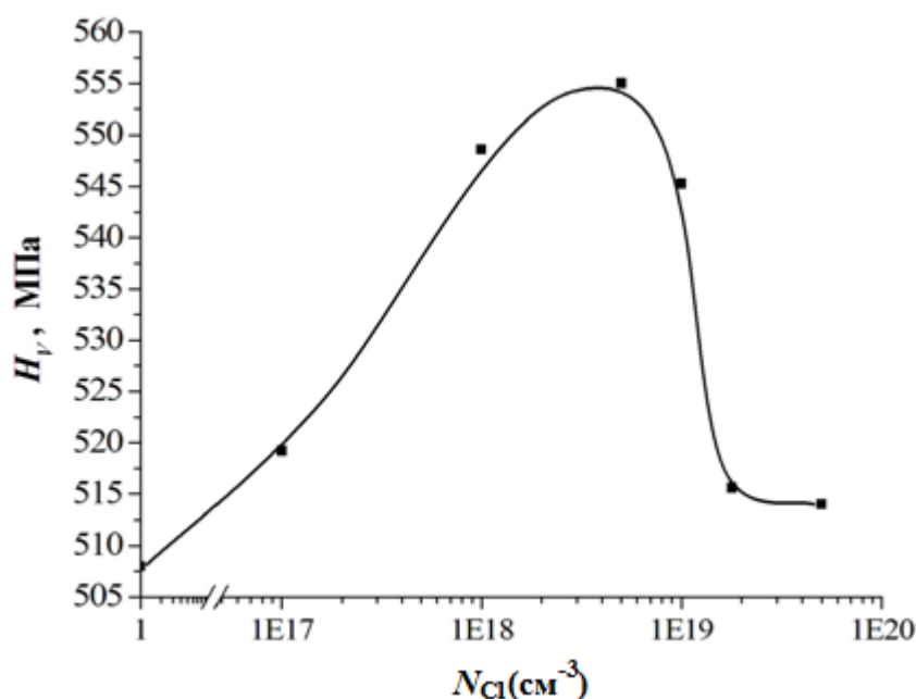
Рис. 1. Залежність мікротвердості монокристалів CdTe від концентрації легуючої домішки Cl
