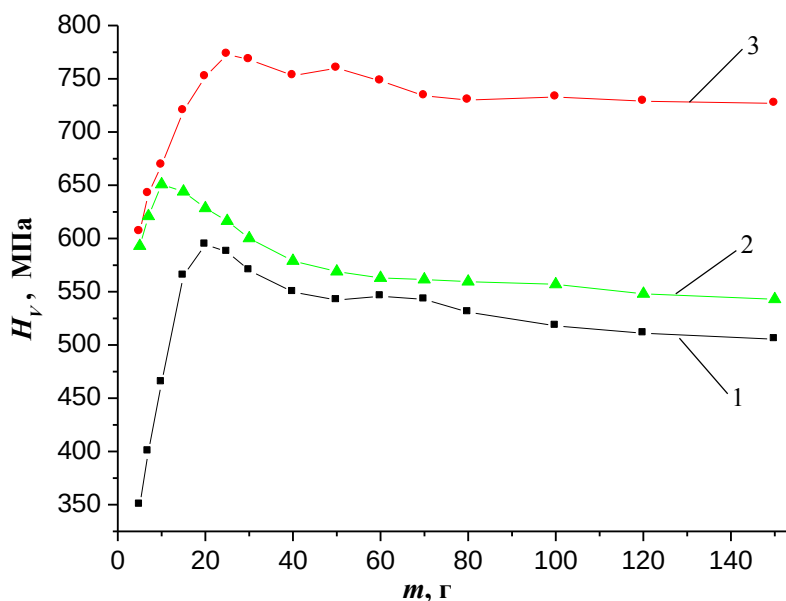
Рис. 1. Мікротвердість монокристалів \text{Cd}_x\text{Zn}_{1-x}\text{Te} : 1 – чистий \text{Cd}_x\text{Zn}_{1-x}\text{Te} ; 2 – \text{Cd}_x\text{Zn}_{1-x}\text{Te} легований хлором 10^{19} \text{ см}^{-3} ; 3 – легований ванадієм 10^{19} \text{ см}^{-3}
