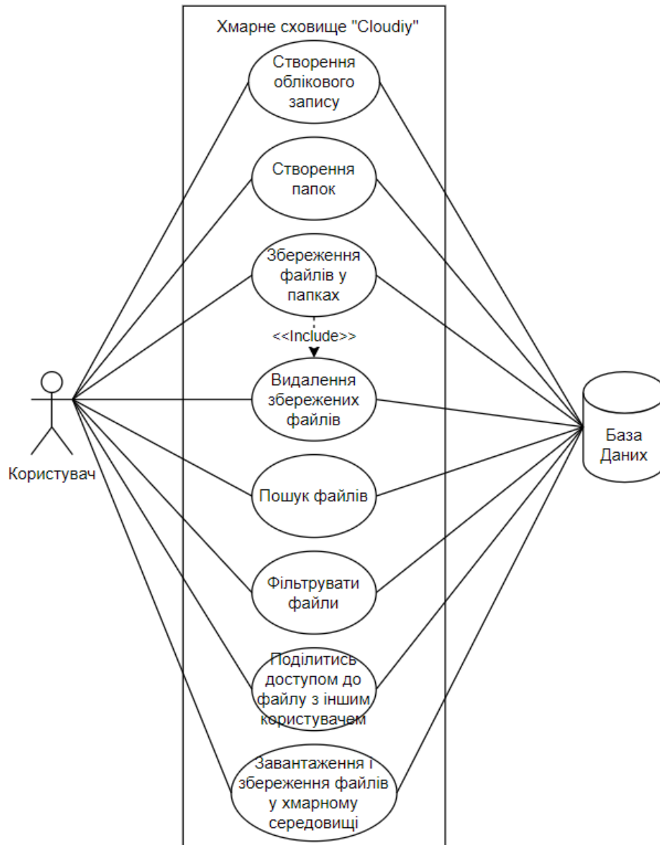
Рис. 1. UML Use Case Diagram додатку
