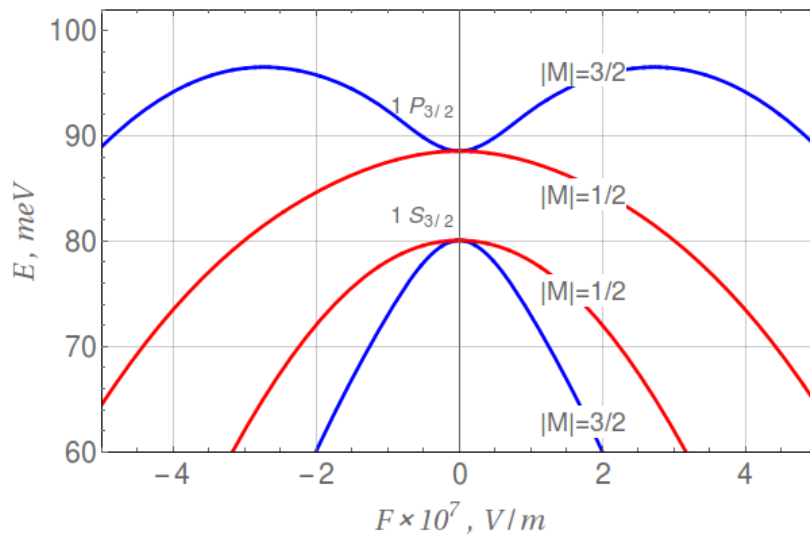
Рисунок 1. Енергії дірки для 1S_{3/2} і 1P_{3/2} станів як функції електричного поля. Радіус КТ - 40 Å.
