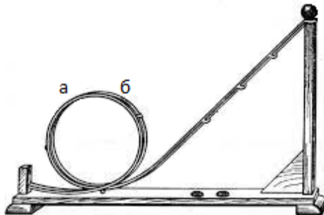
Рис.1. Фотографічне зображення приладу «Мертва петля»
