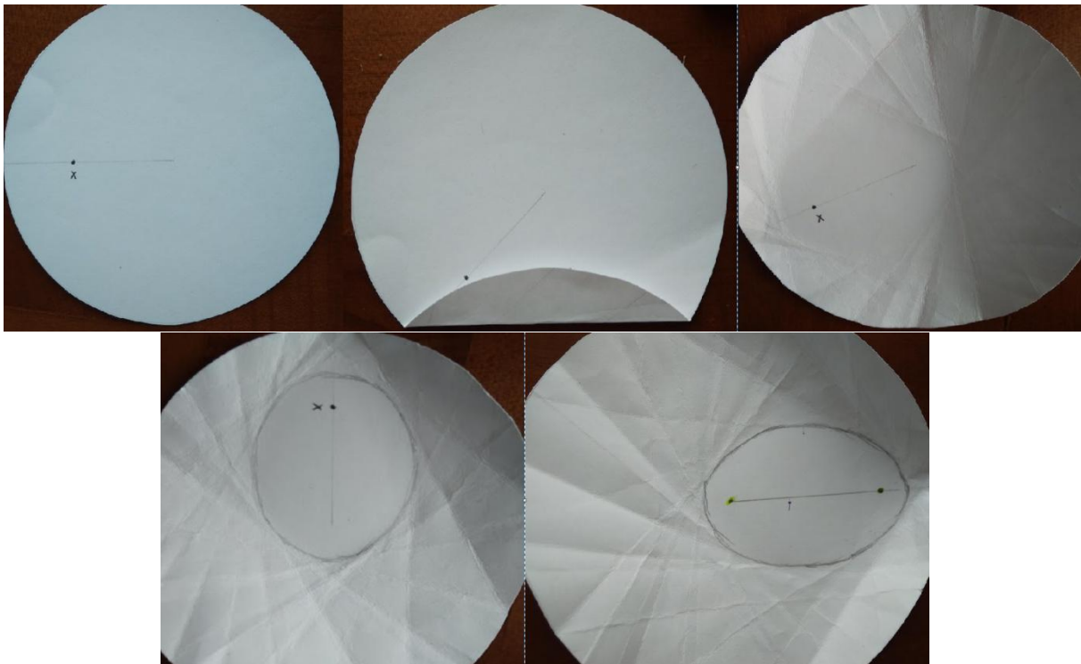
Рис.2. Макет еліпса
