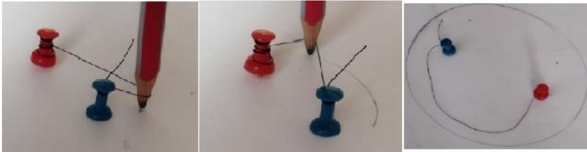
Рис.1. Еліпс
