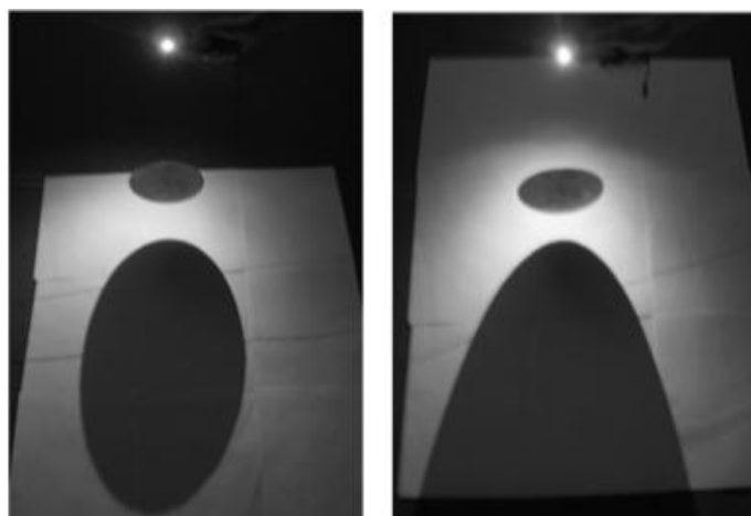
Рис.3. Тіні кола
