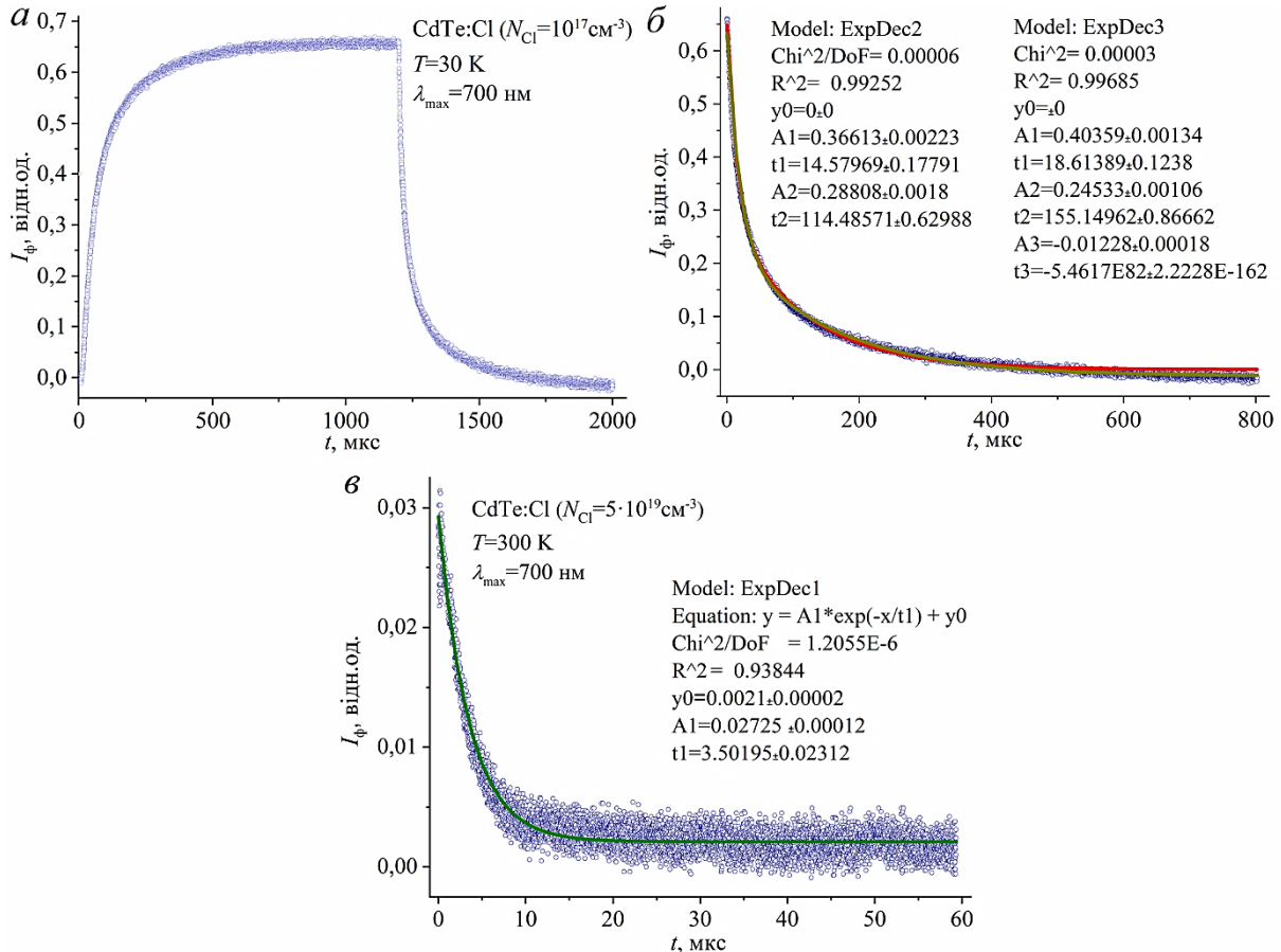
Рис. 1. (а) Типова крива релаксації фотоструму для зразка CdTe:Cl з N_{Cl} = 10^{17} cm^{-3} при T = 30 K . (б) Результат апроксимації спадної ділянки кривої рис. (а) як суми двох (червона лінія) та трьох (жовта лінія) експонент. (в) Представлення спадної ділянки кривої релаксації фотоструму для зразка CdTe:Cl з N_{Cl} = 5 \cdot 10^{19} cm^{-3} при T = 300 K однією експонентою (зелена лінія).
