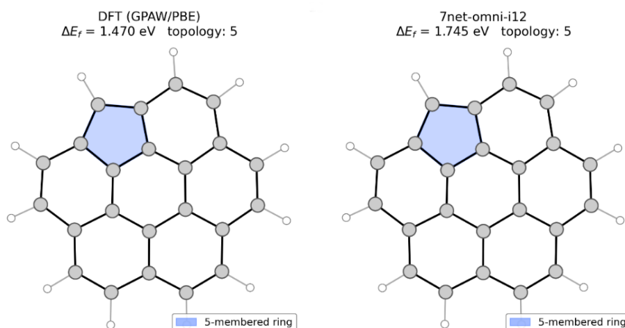
Рис. 1. Структура моновакансії у графеновій квантовій: топологія 5 (одне п'ятичленне кільце). Ліворуч – результат DFT (GPAW/PBE), \Delta E_f = 1.470 eV; праворуч – результат MLIP (7net-omni-i12), \Delta E_f = 1.745 eV. Синім виділено п'ятичленне кільце, що утворюється після релаксації вакансії.
