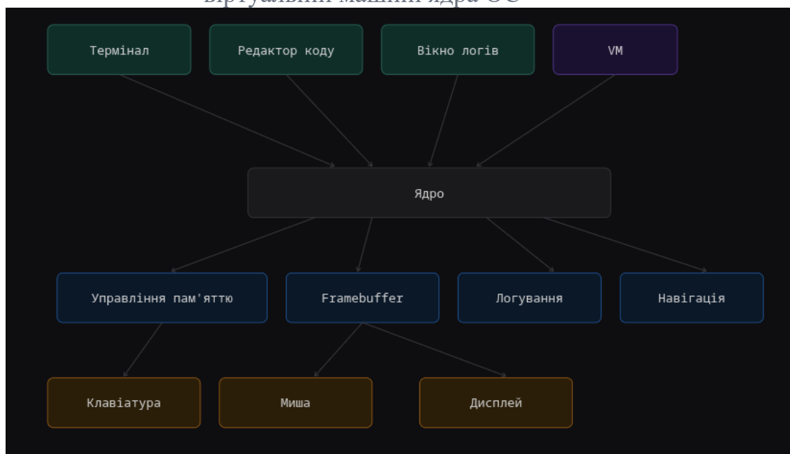
Рис. 2. Структурна діаграма компонентів ядра операційної системи
