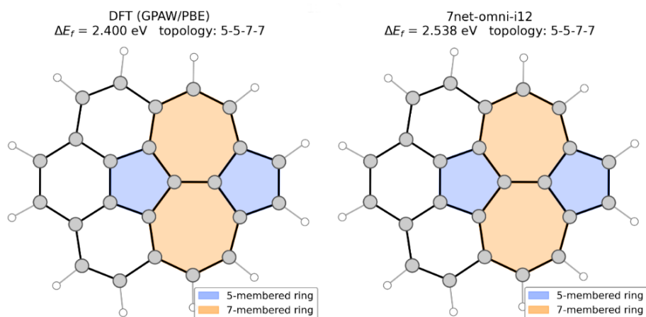
Рис. 2. Структура дефекту Стоуна-Уельса (SW) у графеновій квантовій точці: топологія 5-5-7-7 (два п'ятичленних і два семичленних кільця). Ліворуч – результат DFT (GPAW/PBE), \Delta E_f = 2.400 еВ; праворуч – результат MLIP (7net-omni-i12), \Delta E_f = 2.538 еВ. Синім виділено п'ятичленні кільця, помаранчевим – семичленні.
