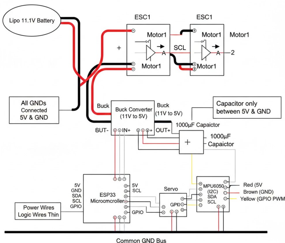
Рис. 2. Електрична схема
