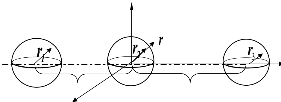
Рис. 1. Модель досліджуваної квантової молекули.
