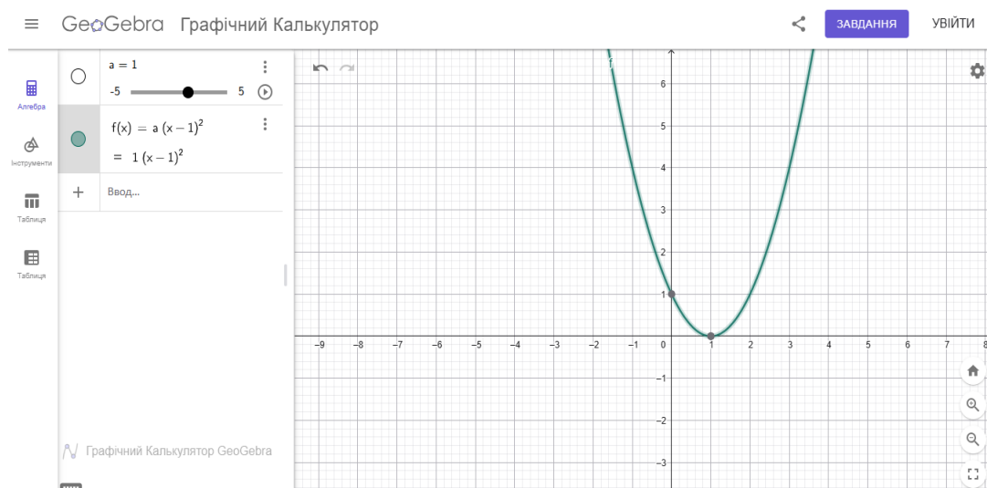
Рис. 1. Графічна інтерпретація функції з параметром
