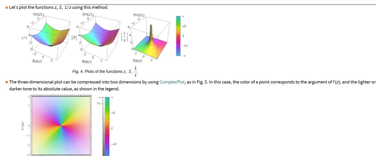
Рис. 3. Візуалізація функцій комплексної змінної в Wolfram Mathematica
