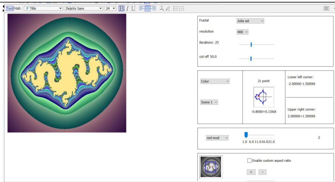
Рис. 2. Графічне зображення ітераційних залежностей Жуліа в Maple.
