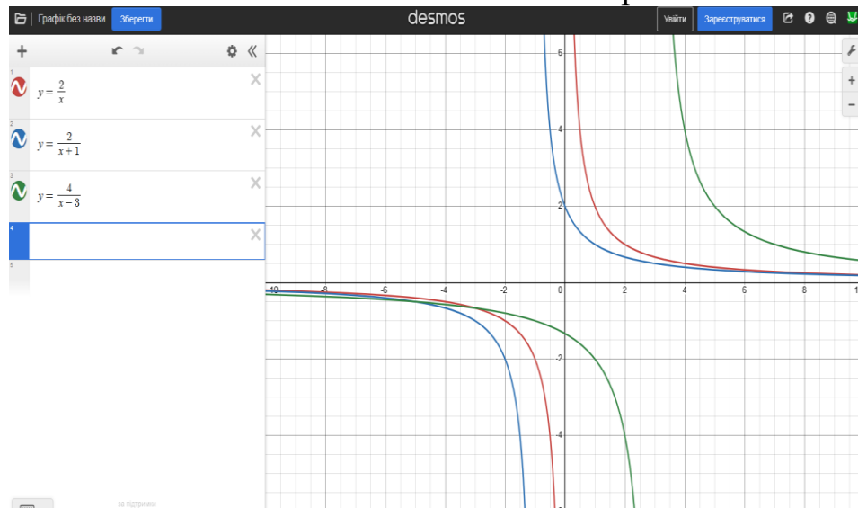
Рис.1. Динамічне дослідження впливу параметра k на розташування віток гіперболи у середовищі Desmos
